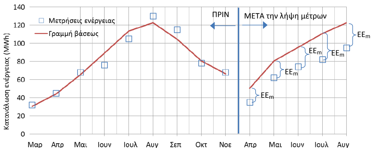
Σχήμα 8.1. : Γραμμή βάσης και εξοικονόμηση ενέργειας
