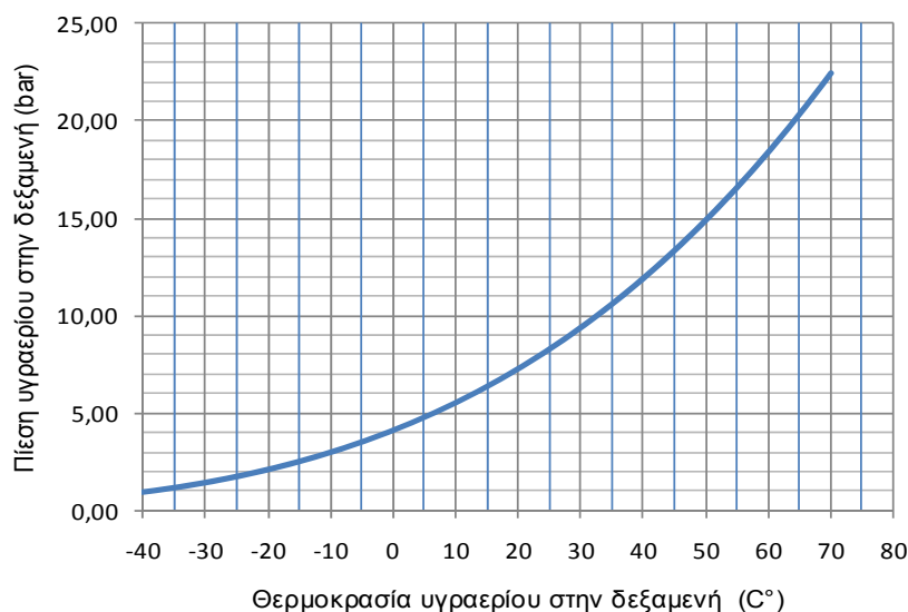
Σχήμα 3.1 Καμπύλη πίεσης – θερμοκρασίας εμπορικού προπανίου σε συνθήκες κορεσμού
